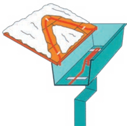
Nel disegno viene mostrato il tracciamento della grondaia, l'ingresso del cavo nel pluviale e il tracciamento della falda del tetto.
